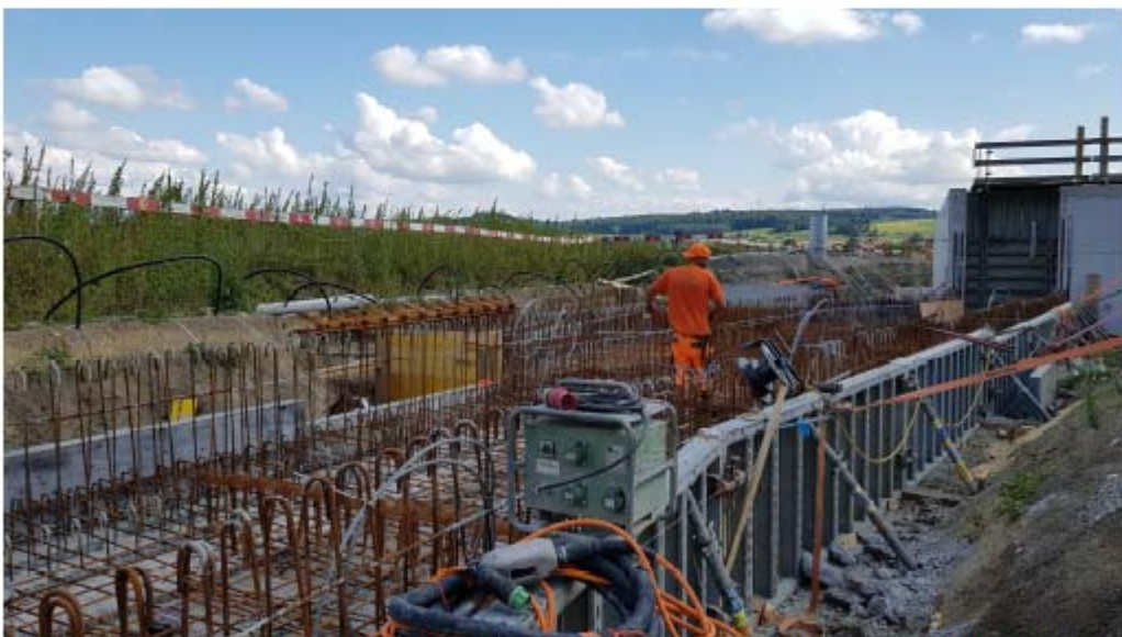
Blick auf den Zuführkanal und Richtung Süden zum Überlauf in die Retentionsfläche
